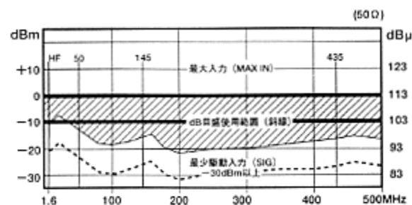
LA-100 周波数対入力特性(参考値) TYP
