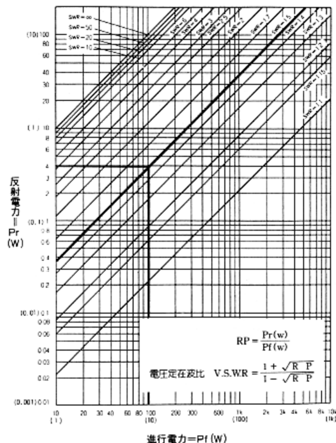
S.W.R.換算表
